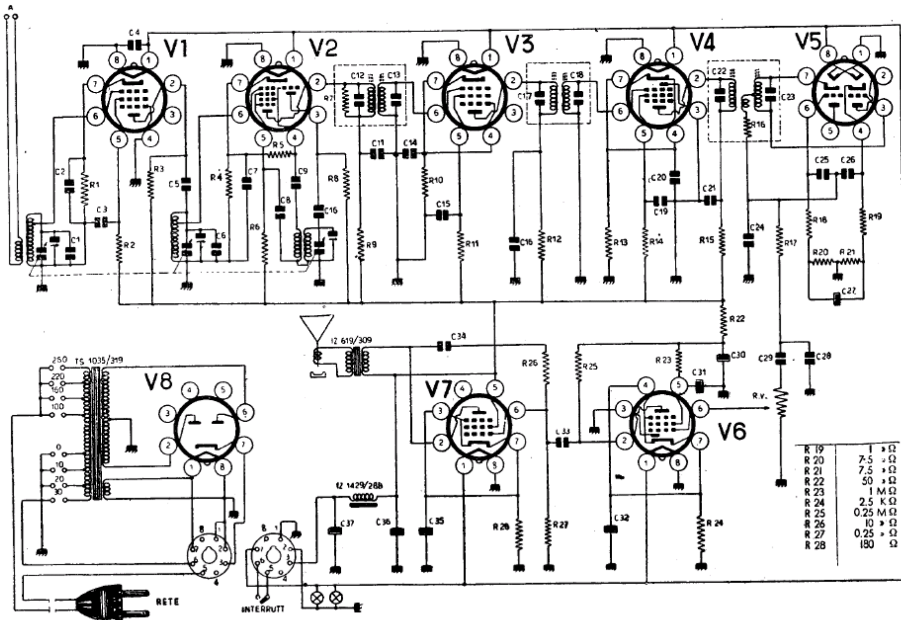
PHONOLA RADIO - Mod. MF 801 - Ricevitore a sola modulazione di frequenza. Gamma 88-108 Mc. Media frequenza 10,7 Mc. V1 amplif. RF, V2 miscelatrice, V3 e V4 amplif. MF, V5 rivelatrice a rapporto, V6 e V7 amplif. BF. Potenza 4 W.
